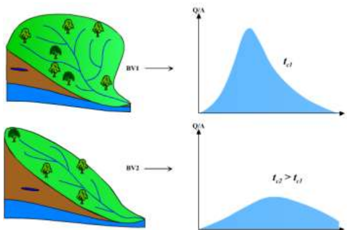
Fig. 9. Influence de la forme du bassin versant sur l'hydrogramme de crue (A. Musy)
