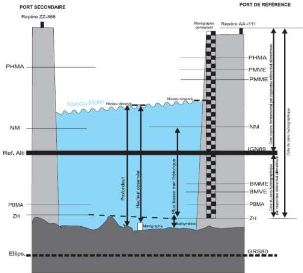
Fig. 94. Schéma récapitulatif des niveaux de marée (cas des marées semi-diurnes)
