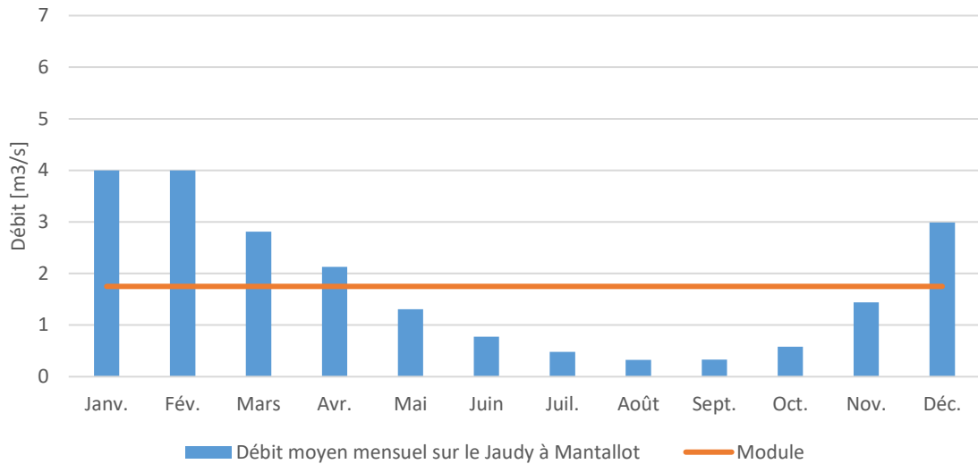
Fig. 88. Débits moyens mensuels et module du Jaudy à Mantallot
