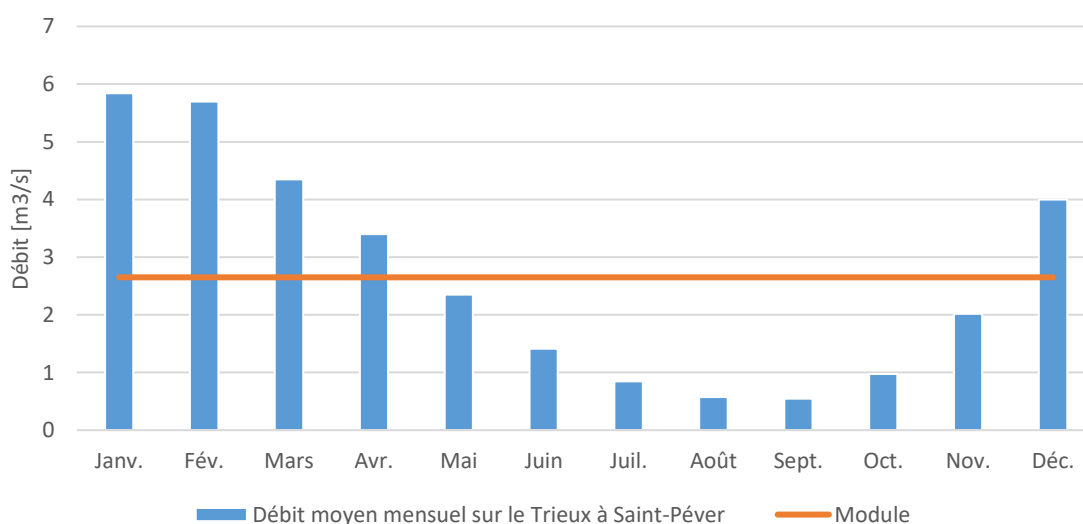
Fig. 87. Débits moyens mensuels et module du Trieux à Saint-Péver
