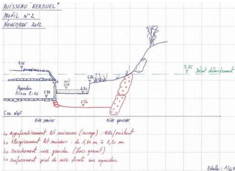
Fig. 62. Exemple du profil existant et du profil projeté du ruisseau du Kerduel
