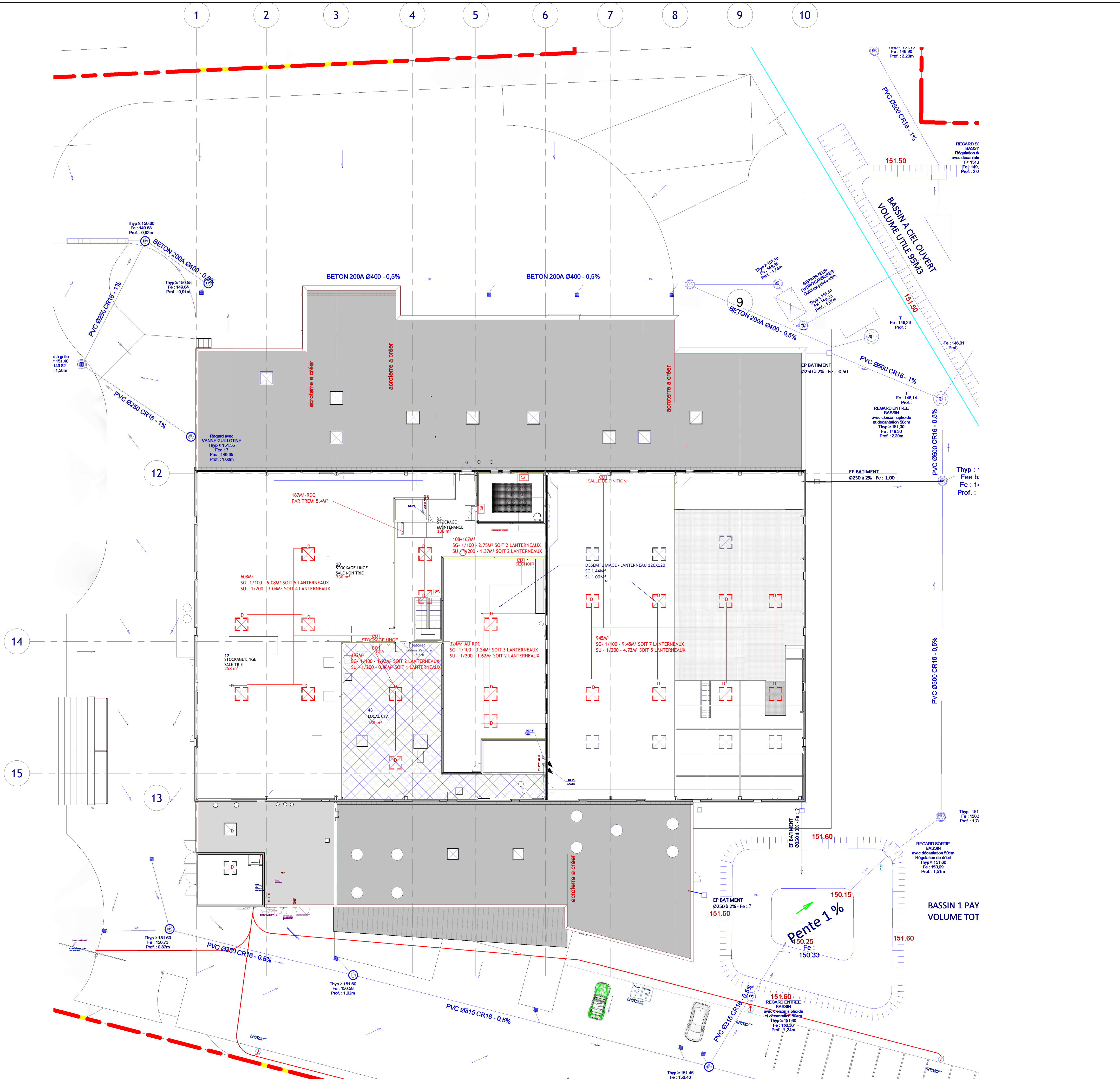
R+1 PROTECTION RISQUE INCENDIE 1 : 200
