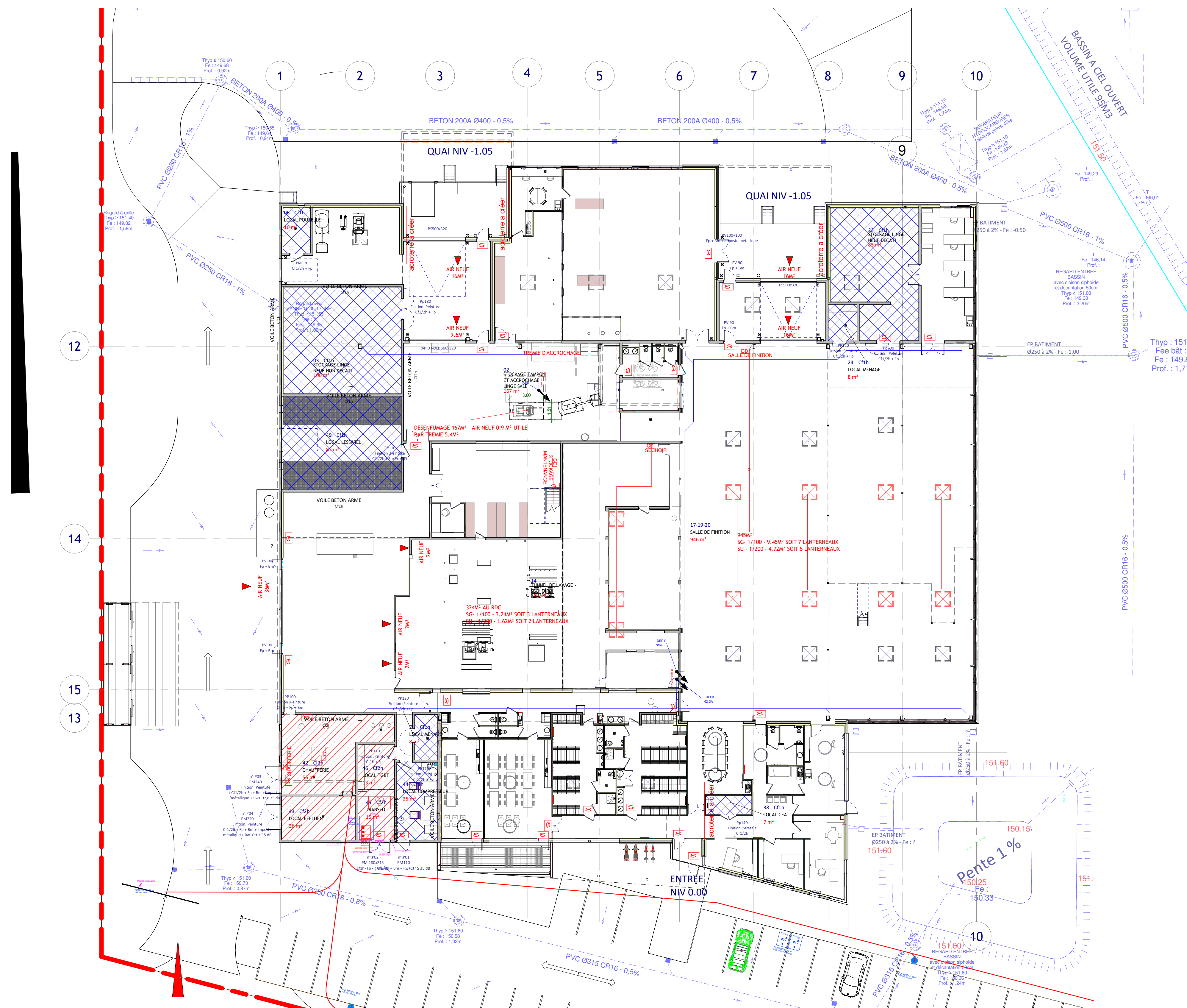
Plan masse 1 : 500
