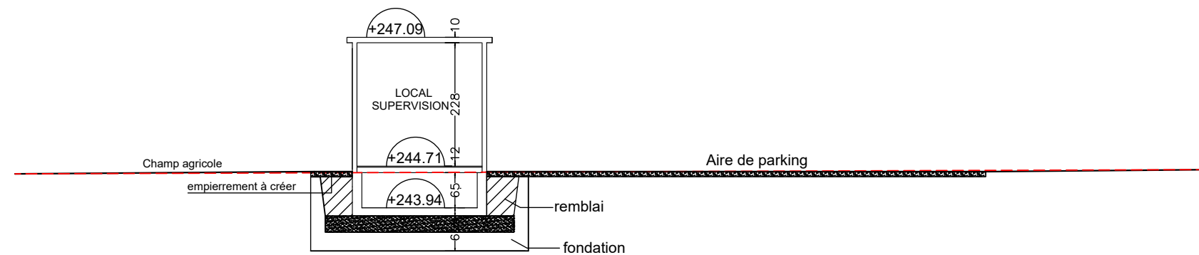
COUPE BB sur Terrain Naturel
